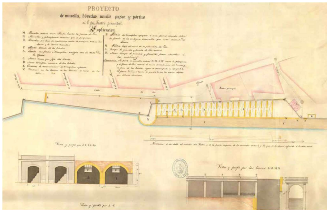
Proyecto de muralla, bóvedas, muelle, paseo y pórtico al Este del Teatro Principal. 1841. La Habana. Ingeniero militar Juan María Muñoz. Archivo General Militar de Madrid (ver enlace).
